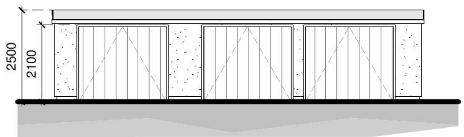
East 1 : 100
